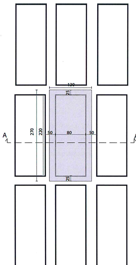
Figura 1 - Schema fosse di inumazione - Pianta
