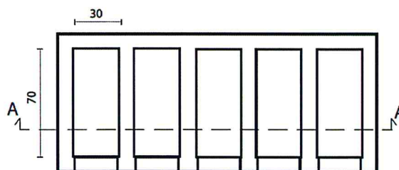
Figura 4 - Schema ossari - sezione
